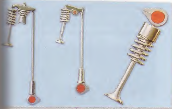
Balancines activados en diferentes formas
